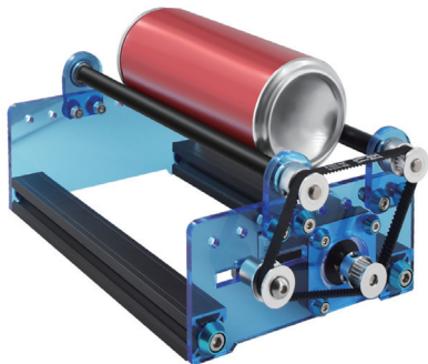
Rotate Module
