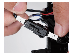
E(3PIN)→Flammenwächter-Signalkabel
