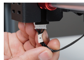
Y(4PIN)→Achsen-Schrittmotorkabel
