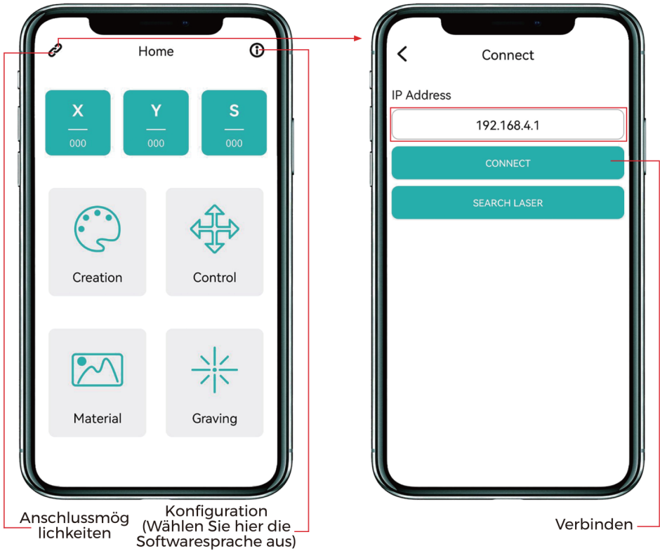
APP-Hauptschnittstelle
