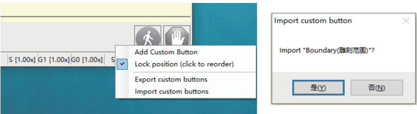
Abbildung 5.2 Hinzufügen
