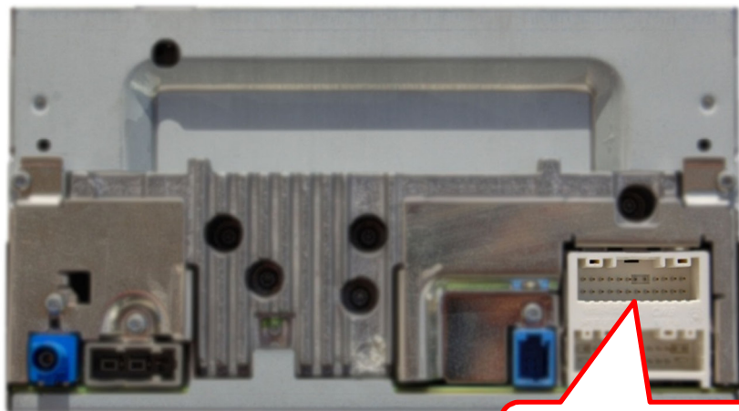
24 PIN ГНЕЗДО ДЛЯ ПОДКЛЮЧЕНИЯ КАМЕРЫ ЗАДНЕГО ВИДА
