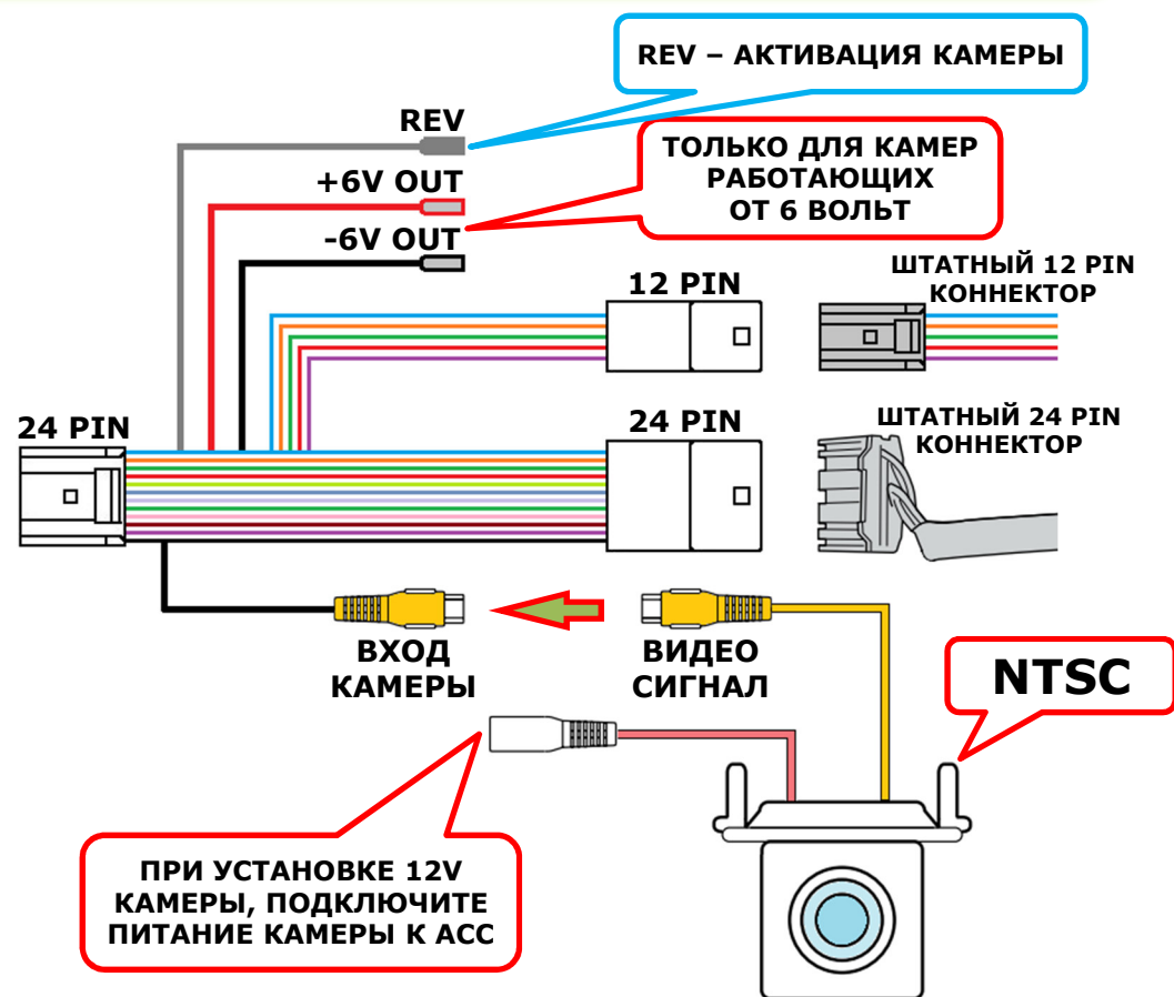
24 PIN ГНЕЗДО ДЛЯ ПОДКЛЮЧЕНИЯ КАМЕРЫ ЗАДНЕГО ВИДА
