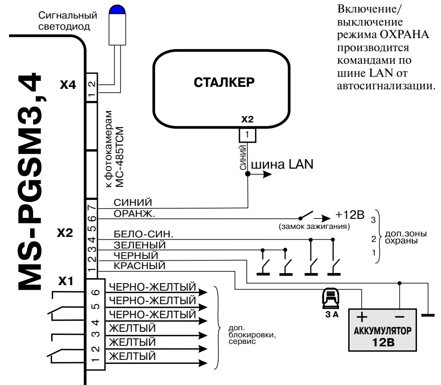
Рис. 17. Подключение GSM-автопейджера MS-PGSM2 по шине LAN
