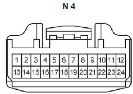
Вид спереди
